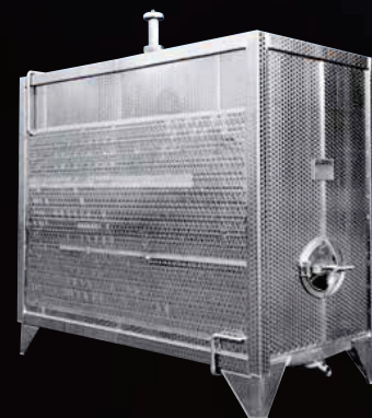
Serbatoio Compatank con pareti termocondizionate con Termostar
