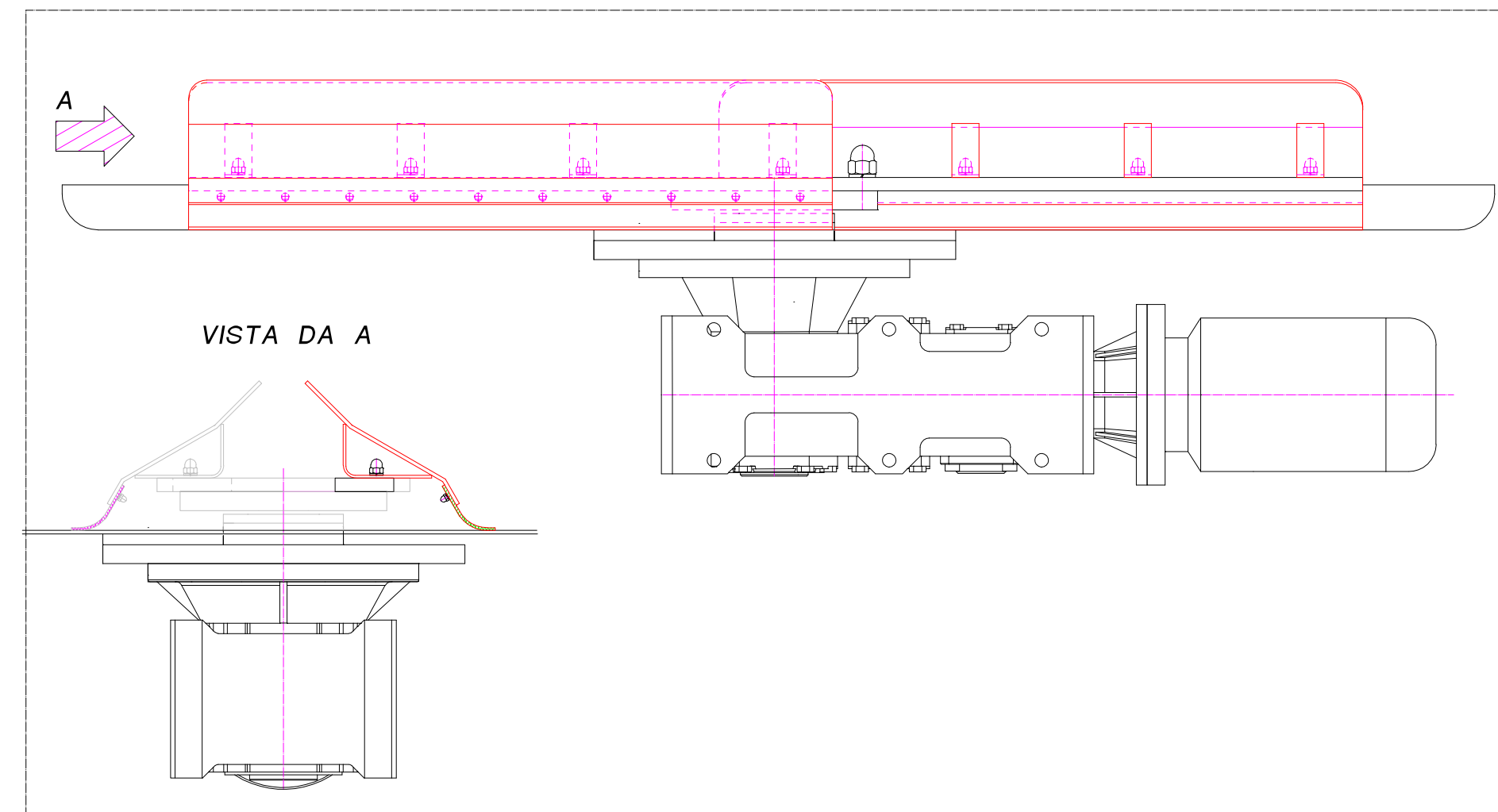
PALA DI ESTRAZIONE CON SISTEMA SMONTABILE DI BATONAGE E SCARICO VINACCIOLI
