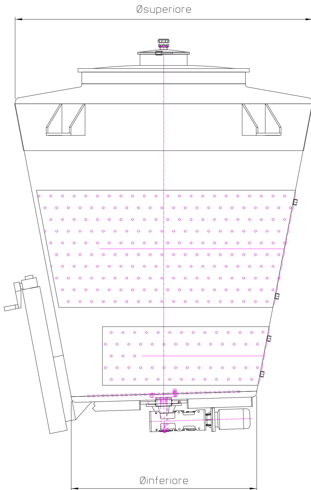
MODELLO CON STAFFE DI SUPPORTO SUPERIORI
