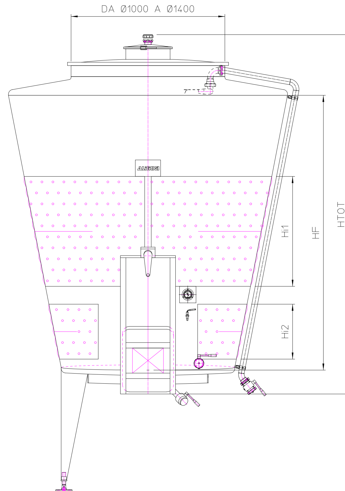
PALA DI ESTRAZIONE PREDISPOSTA PER MONTAGGIO SISTEMA DI BATONAGE E SCARICO VINACCIOLI
