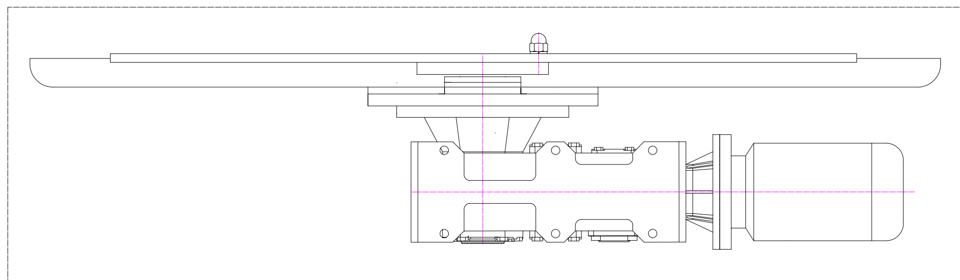
PALA DI ESTRAZIONE PREDISPOSTA PER MONTAGGIO SISTEMA DI BATONAGE E SCARICO VINACCIOLI
