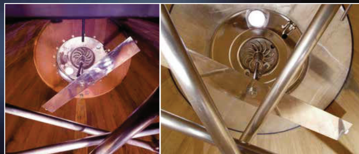
Vista dall'interno di tini di legno con pala autorotante brevettata e pali rompiscappello per fare la follatura e il délestage
