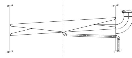
Fondo conico con il sistema di controfondo brevettato Albrigi Superbottom inclinato del 3% per sfiatare tutta l'aria
