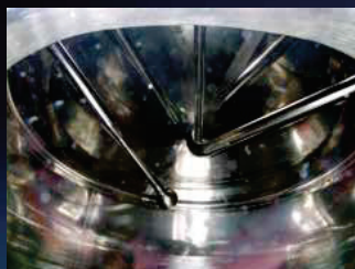
Fondo e contro fondo brevetto Albrigi Superbottom con sfera di lavaggio Sprayball
