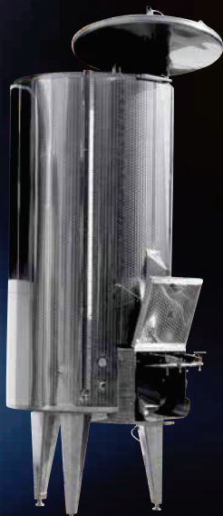
Variotank isolato Isofix con intercapedine di condizionamento Termostar per criomacerazione
